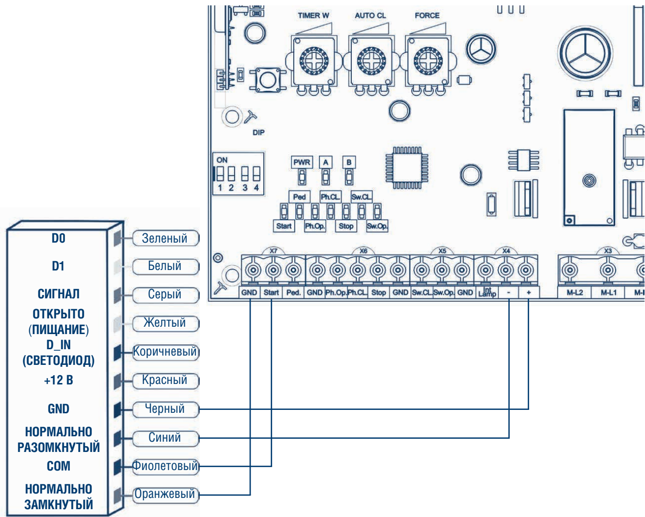
Рис. 3.3. Подключение внешнего считывателя
